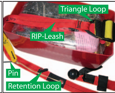
RIP-Leash
